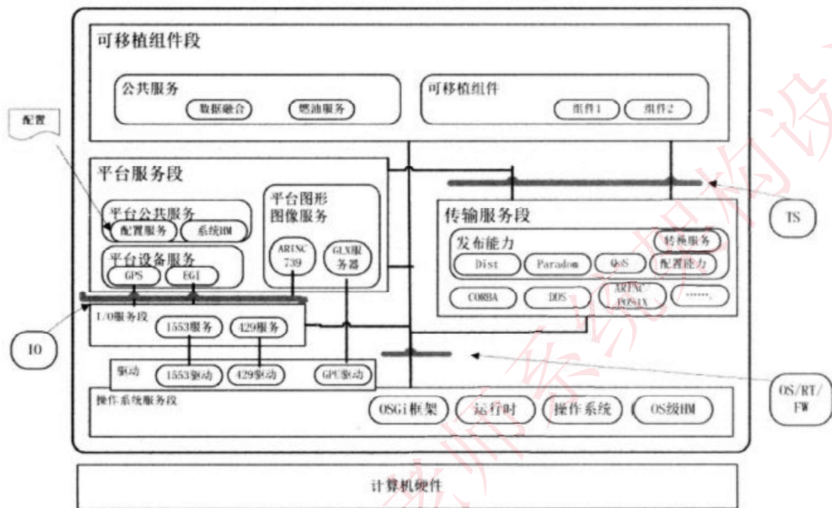
图 3-1 FACE 架构
